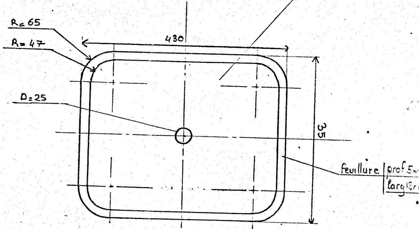
COUVERCLE COFFRE POSTE AV
