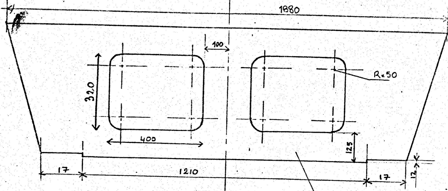
SUPPORT DE COUCHETTES POSTE AV ELEMENT AR
